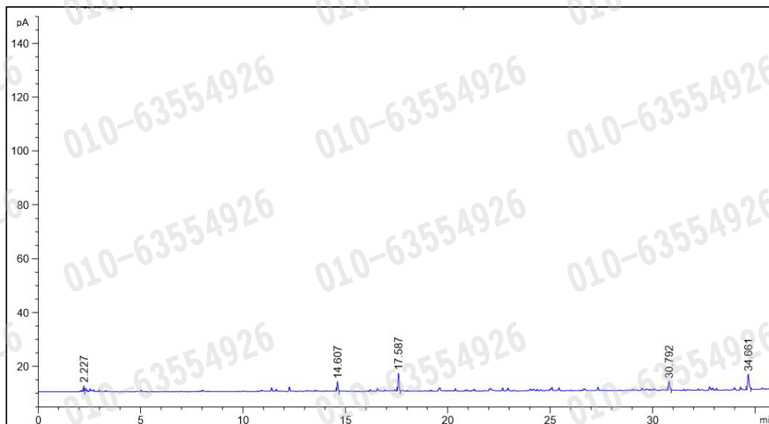
本底谱图
