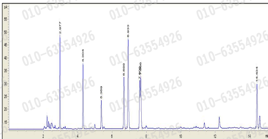
加标谱图
